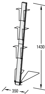
PG-3 3 lattice trays DIN A4
