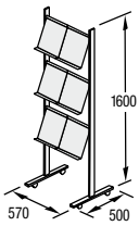
P-6 6 shelves A4
