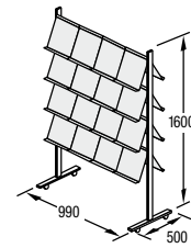
P-32 32 shelves A4
