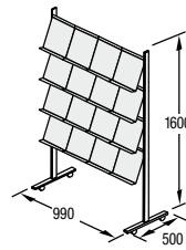
P-16 16 shelves A4
